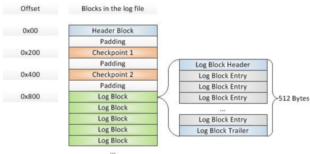
Abbildung 77 – Struktur der Transaction-Logs
